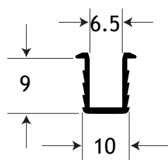
Sliding Door Upper Track
